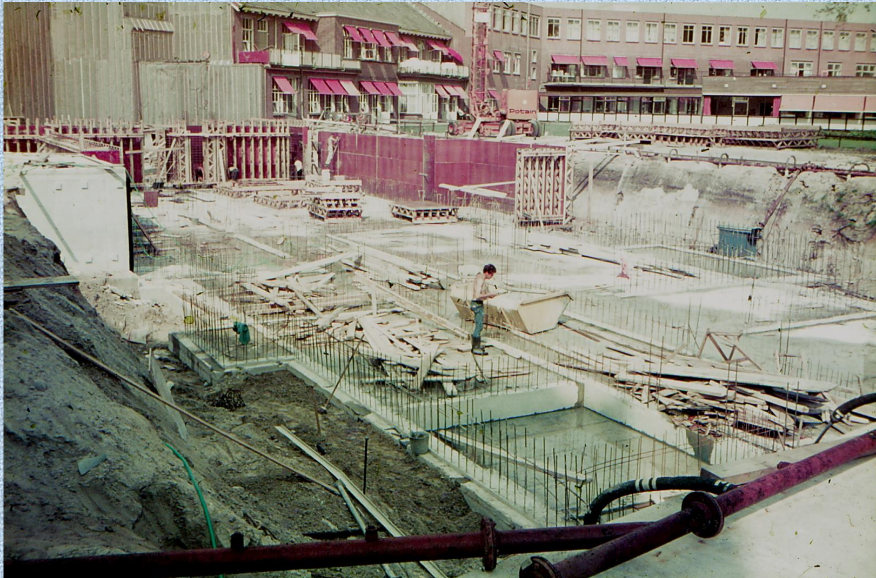
De kelder onder het beddenhuis (Gebouw B)
