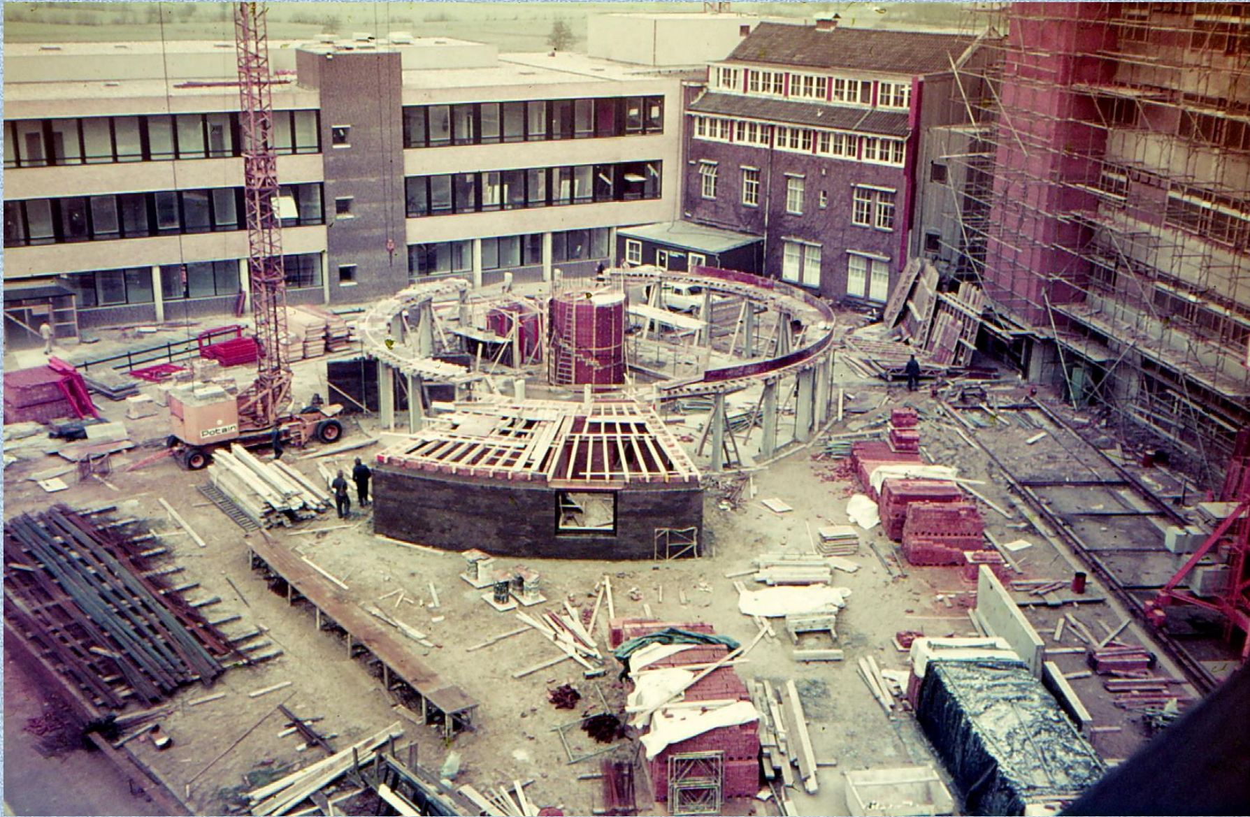
De nieuwe receptie krijgt vorm. Rechts de liftschacht voor het beddenhuis, middenrechts nog een deel van het oude gebouw
